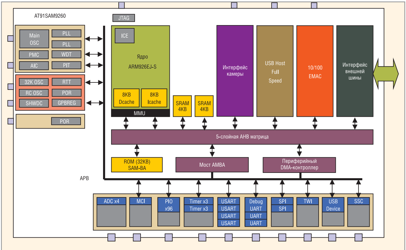
Рис. 2. Структурная схема микроконтроллера AT91SAM9261
