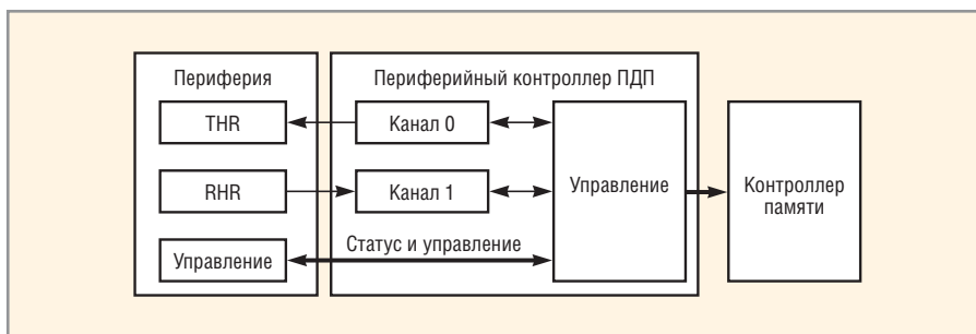
Рис. 1. Структура многоканального контроллера PDC
