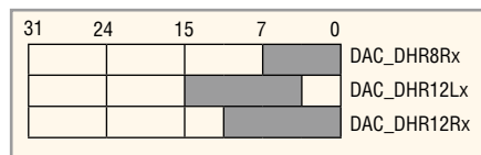
Рис. 2. Способы загрузки регистра DAC_DORx в режиме одиночных каналов
