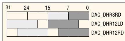
Рис. 3. Способы загрузки регистра DAC_DORx в режиме двоеканальных
