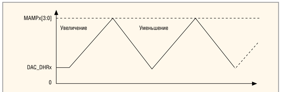
Рис. 6. Осциллограмма генерации шума
