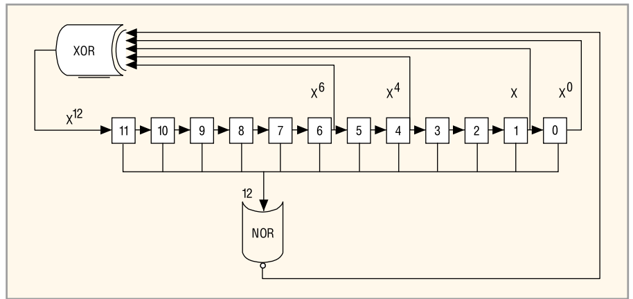
Рис. 4. Алгоритм вычисления сигнала шума
